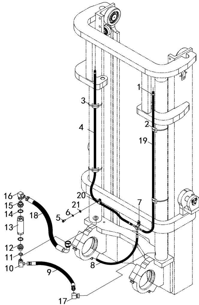
图 6 管路系统 Fig.6 Lifting oil circuit
