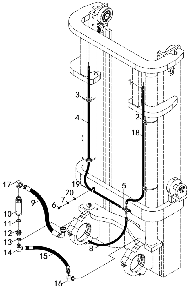
图 22 管路系统 Fig.22 Lifting oil circuit
