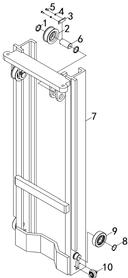
图9 内门架 Fig.9 Inside mast
