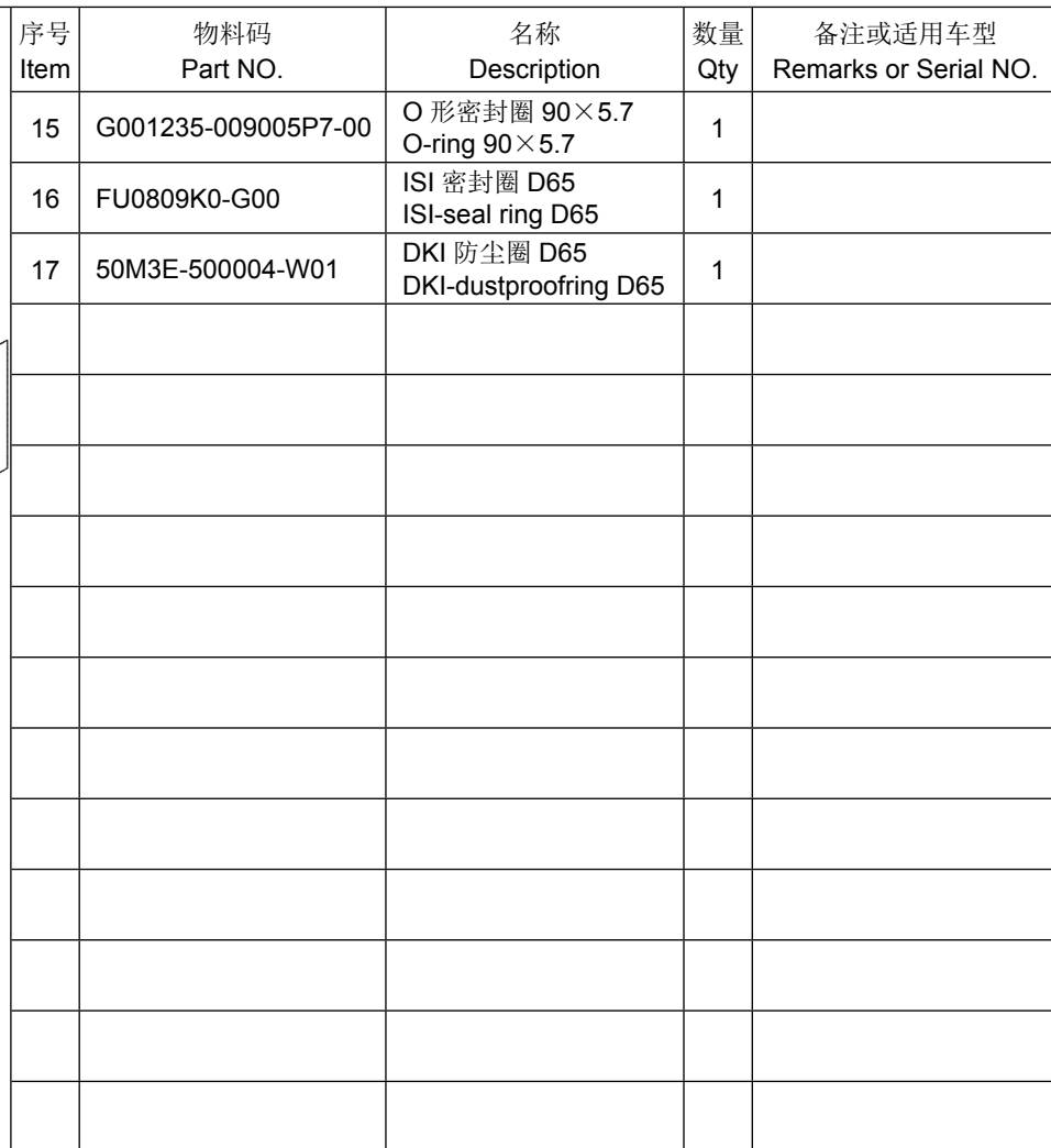
XA 系列 XA Series 2 级门架 SIMPLEX 7t
