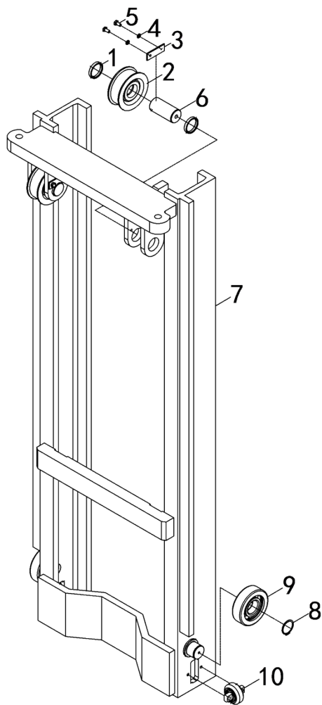
图2 内门架 Fig.2 Inside mast
