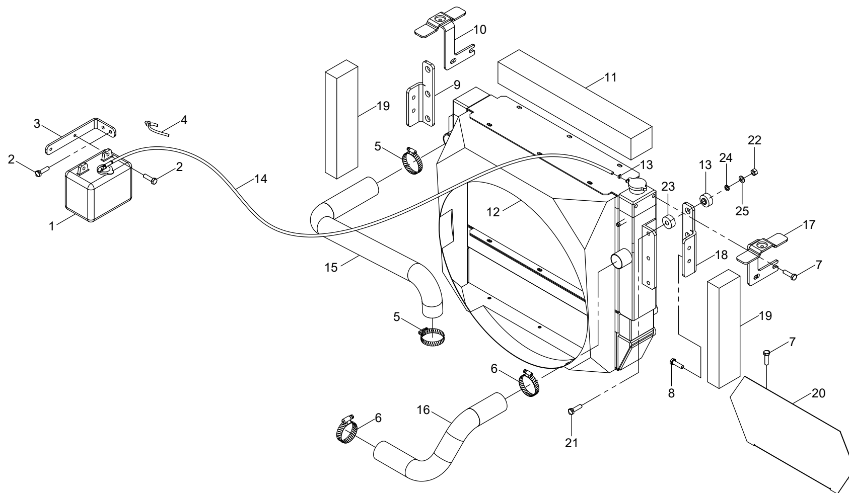
图 10 冷却系统 Fig.10 Cooling system
