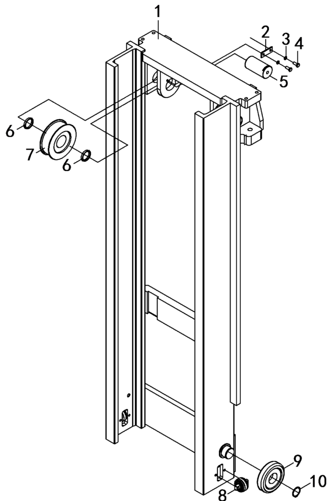
图 25 内门架 Fig.25 Inside mast
