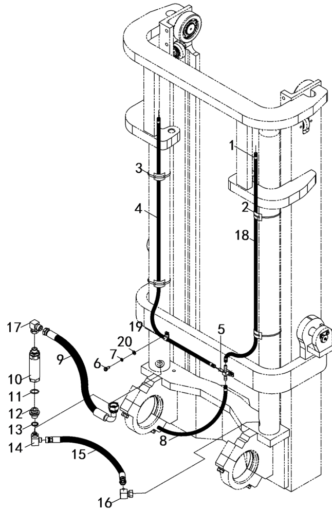
图 29 管路系统 Fig.29 Lifting oil circuit
